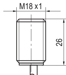
Габаритный чертеж
